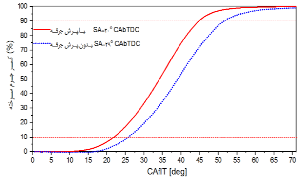
شکل ۶: تغییرات کسر جرم سوخته بر حسب زاویه لنگ در حالت با پرش جرکه و بدون پرش جرکه
