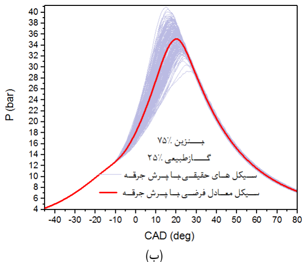
شکل ۲: تغییرات فشار بر حسب زاویه لنگ چرخه‌های حقیقی و چرخه معادل فرضی در شرایط: (الف) بدون پرش جرقه (ب) با پرش جرقه
