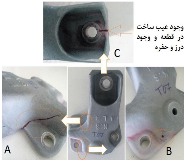
شکل ۶: ترک‌های ایجاد شده پس از آزمون خستگی
