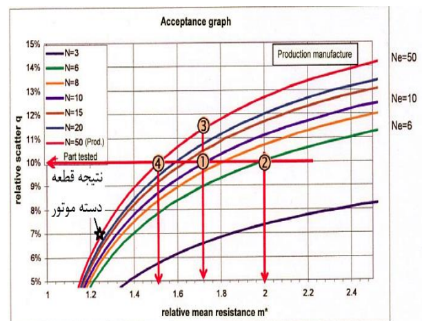
شکل ۵: نتیجه آزمون خستگی مرحله اول پایه دسته موتور آلومینیومی در نمودار خستگی مرجع
