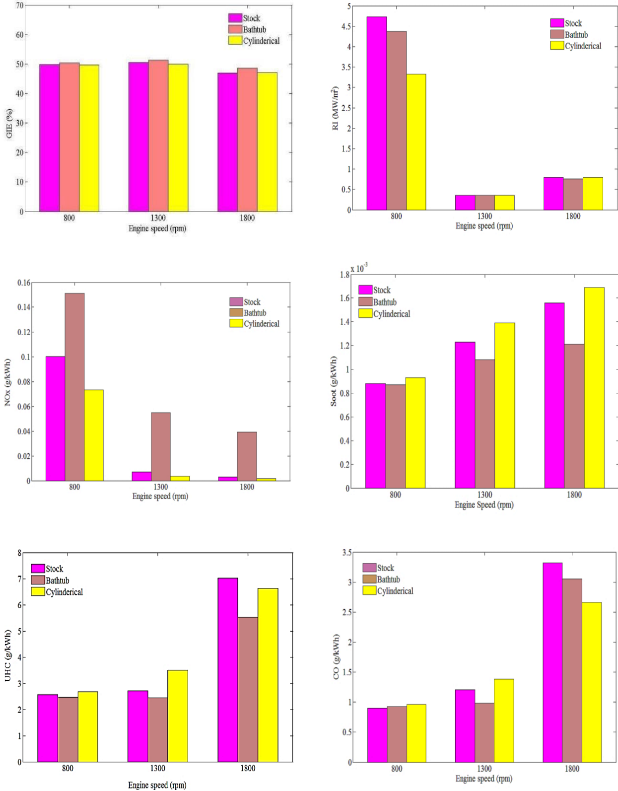
شکل ۶: مقایسه نتایج عملکرد و آلاینده‌گی برای سه هندسه مختلف در سرعت‌های مختلف در احتراق RCCI گاز طبیعی- دیزل در IMEP 9
