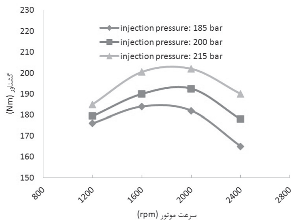
شکل ۷ گشتاور برحسب سرعت موتور برای سوخت B20 به ازای مقادیر مختلف فشار پاشش
