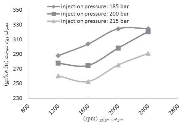
شکل ۹ مصرف ویژه سوخت برحسب سرعت موتور برای سوخت B۱۰۰ به ازای مقادیر مختلف فشار پاشش
