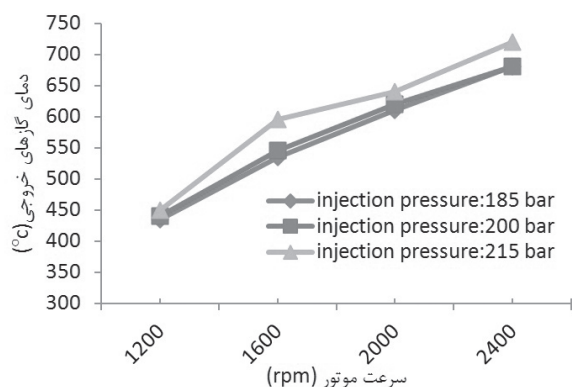
شکل ۱۰ دمای گازهای خروجی از مجرای دود برحسب سرعت موتور برای سوخت B۲۰ به ازای مقادیر مختلف فشار پاشش
