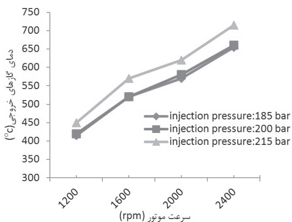
شکل ۱۱ دمای گازهای خروجی از مجرای دود برحسب سرعت موتور برای سوخت B۴۰ به ازای مقادیر مختلف فشار پاشش
