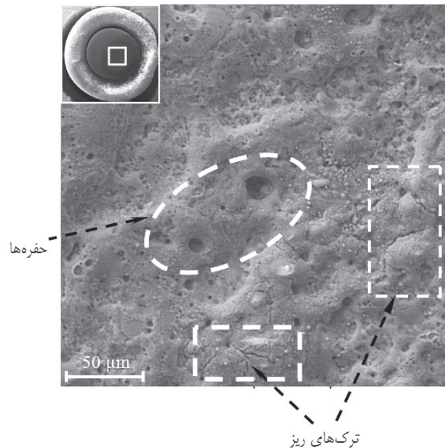
شکل ۱۷ حفرة ها و ترک سطح الکترود مرکزی شمع نوع سوم بعد از ۲۰۰ ساعت کارکرد در آزمون دوام (استوانه شماره ۲)
