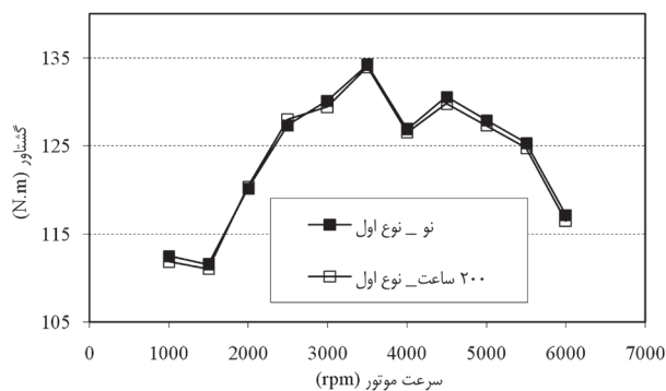
شکل ۲۳ گشتاور موتور با استفاده از شمع‌های نو و کارکرده نوع اول در هنگام کارکرد موتور با سوخت گاز طبیعی در شرایط بار کامل
