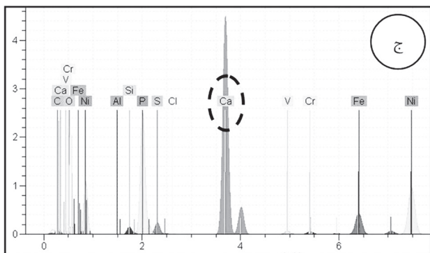
شکل ۱۸ الف و ب) مواد مذاب و متخلخل ناشی از جرقه جانبی. ج) بررسی مواد موجود در سطح کناری الکترود مرکزی شمع نوع سوم بعد از ۲۰۰ ساعت کارکرد در آزمون دوام (استوانه شماره ۲)
