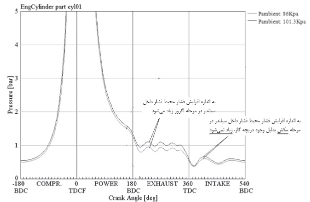
شکل ۴ اثر تغییر فشار محیط بر تغییر فشار ورودی و خروجی
