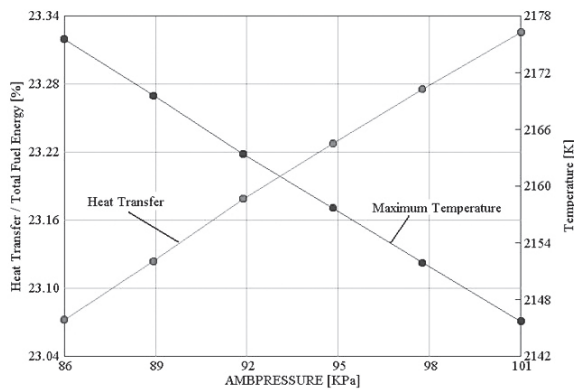
شکل ۶ میزان انتقال حرارت و دمای بیشینه با تغییر فشار محیط ۲-۲۰۰۰ بار
