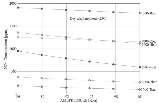
شکل ۷ اثر تغییر فشار محیط بر میزان آلایندگی اکسیدهای نیتروژن
