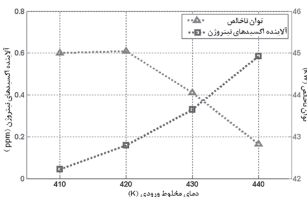
شکل ۷ میزان تولید توان و آلایندگی اکسیدهای نیتروژن در شرایط دمایی ورودی مختلف
