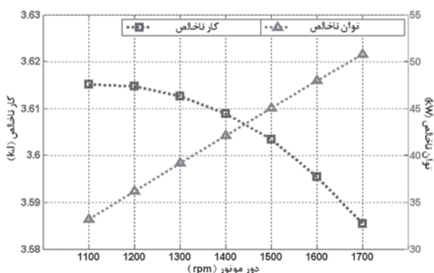
شکل ۱۴ تولید توان و کار در دورهای مختلف موتور
