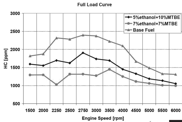
شکل ۹ تغییرات آلایند هیدروکربن‌های نسوخته برحسب دور
