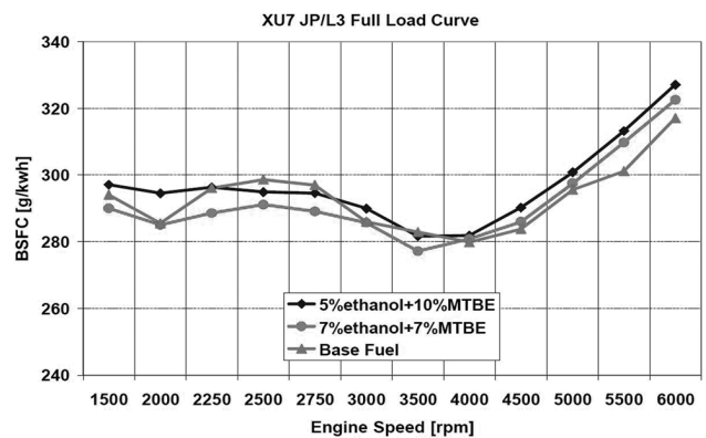
شکل ۶ تغییرات مصرف سوخت ویژه ترمزی به صورت تابعی از سرعت دورانی موتور
