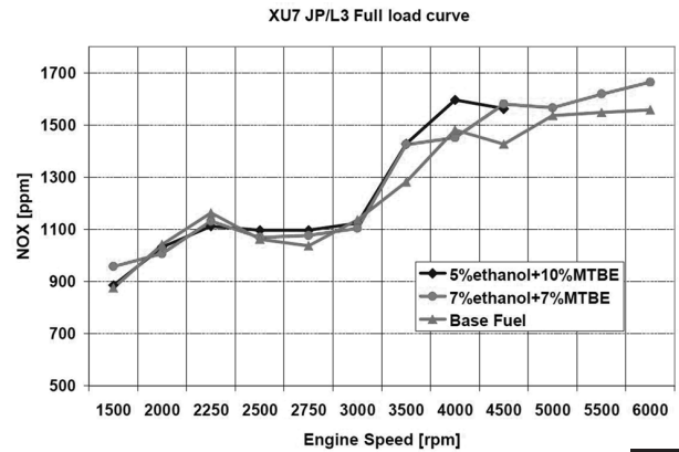
شکل ۸ تغییرات آلایند اکسیدهای نیتروژن برحسب دور برای سوخت‌های مورد استفاده
