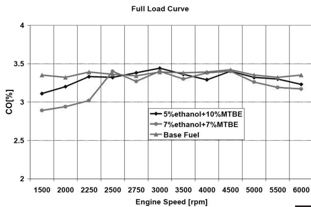
شکل ۷ تغییرات آلایندة مونوکسیدکربن نسبت به تغییر سرعت موتور در وضعیت بار کامل برای سوخت‌های مختلف
